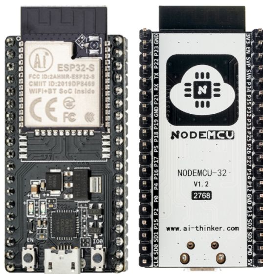
图 4.1 NodeMCU-32S_v1.2 板载 CP2102 外观图(图片及丝印仅供参考，以实物为准)
