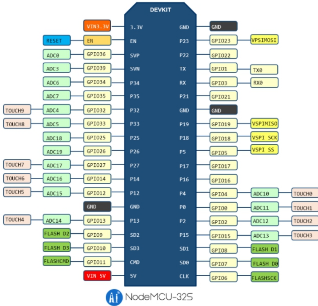
图 7 开发板管脚示意图
